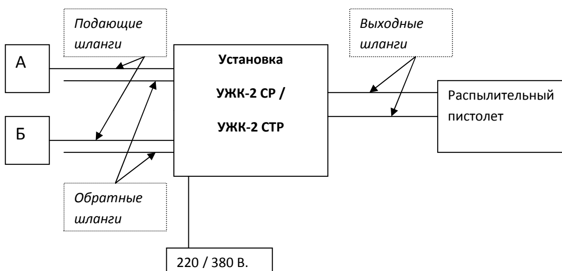
Рис.1 Схема подключения установки
