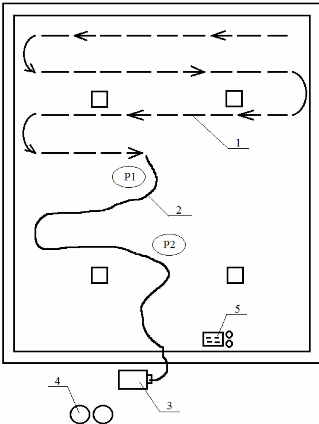
Рис. 1А. Схема организации рабочего места при устройстве гидроизоляции из жидкой резины «СBS».
